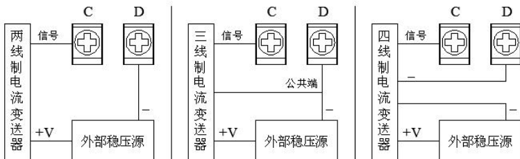
变送器接线方式 (外接稳压源)
