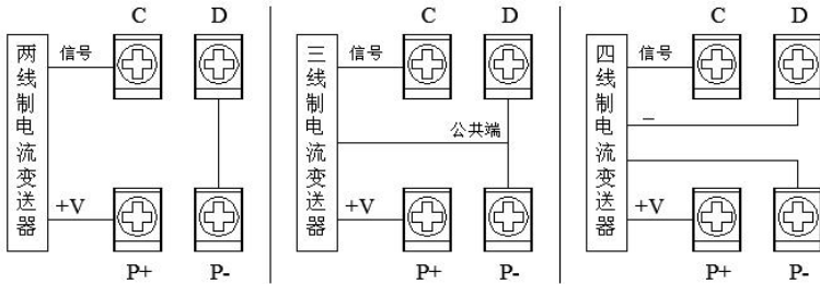
变送器接线方式 (仪表供电)
