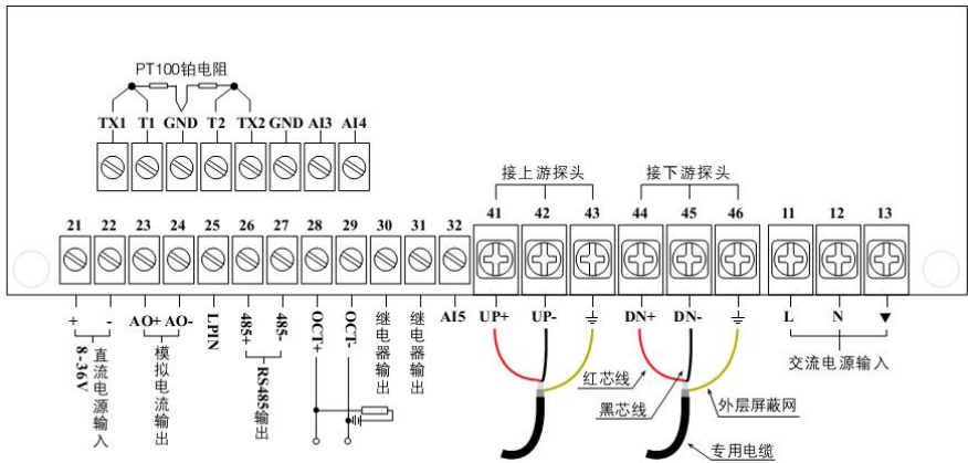
18 版主板接线图
